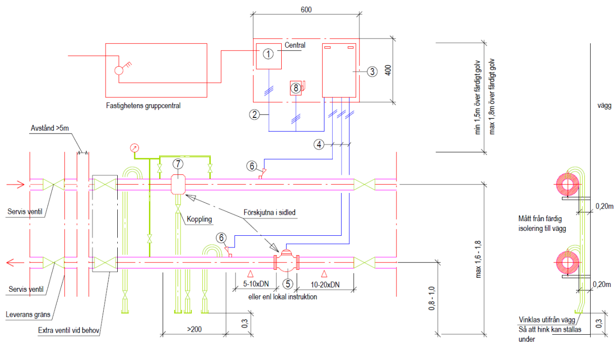
Fig.4 Typritning mätplatsen
