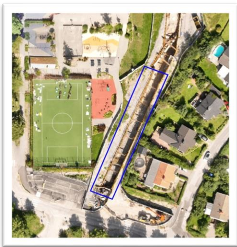
Figur 1: Installation av ledningar.
